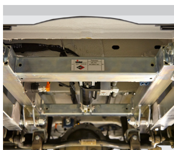
Hydraulische Achsblockierung
